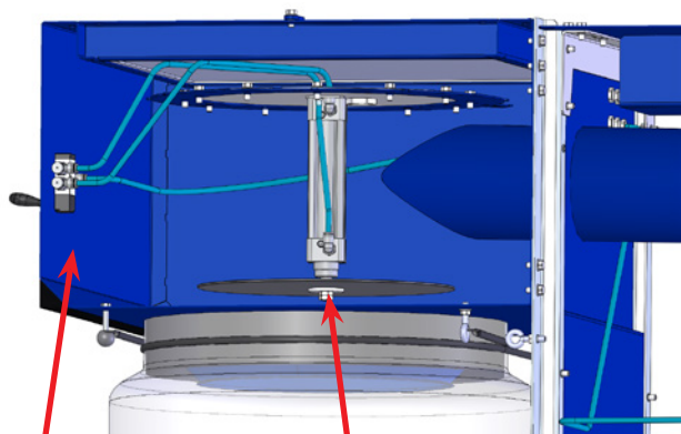
Interrupteur pour vanne de matériau (peut être accessoirisé)
