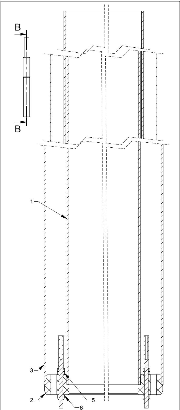
SECTION B-B (1 : 2)
