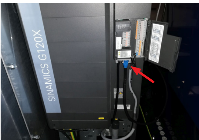
6 - Datakabeln kopplas bort från frekvensomvandlaren - illustreras här på G120X-omvandlaren
