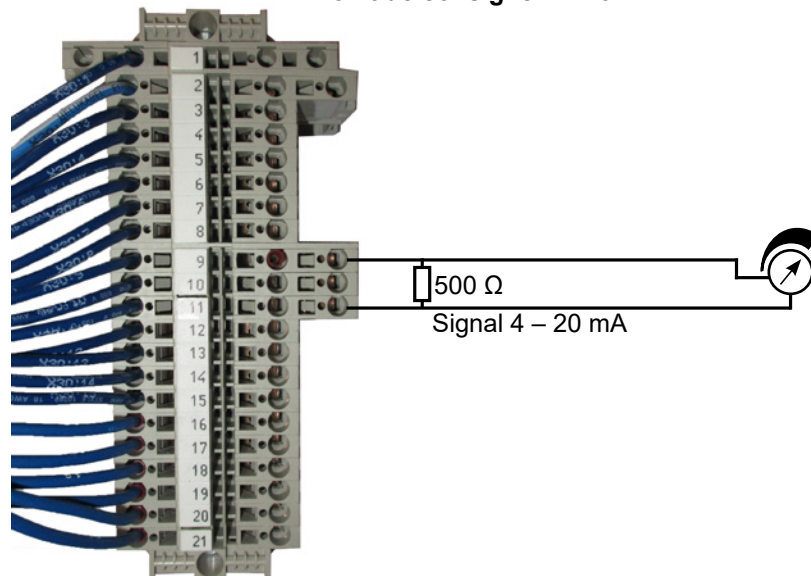
Point de consigne 4 – 20 mA
