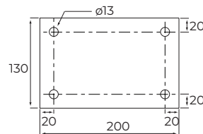
KM 130 – KM 180 Fußplatte
