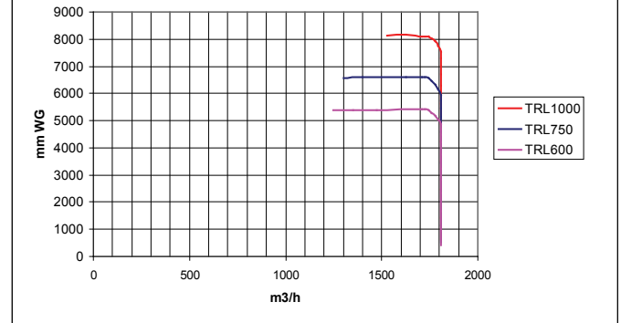
Leistungskurve für TRL600 - 1000 mit Luftregulierung für OK160:
