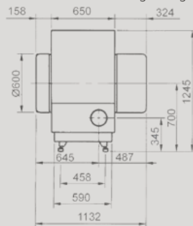
MultiAir 1055 TR med regulering
