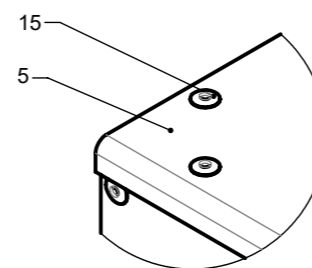
DETAIL D (1 : 2)
