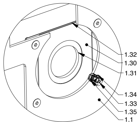
DETAIL D (1 : 3)
