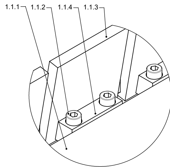
DETAIL B (1 : 2)
