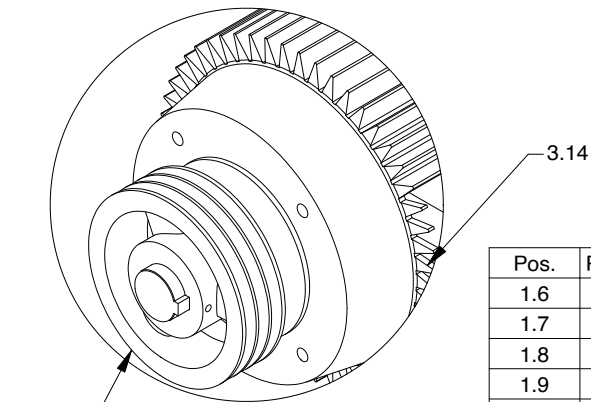
DETAIL D (1 : 5)
