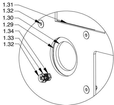
DETAIL D (1 : 3)
