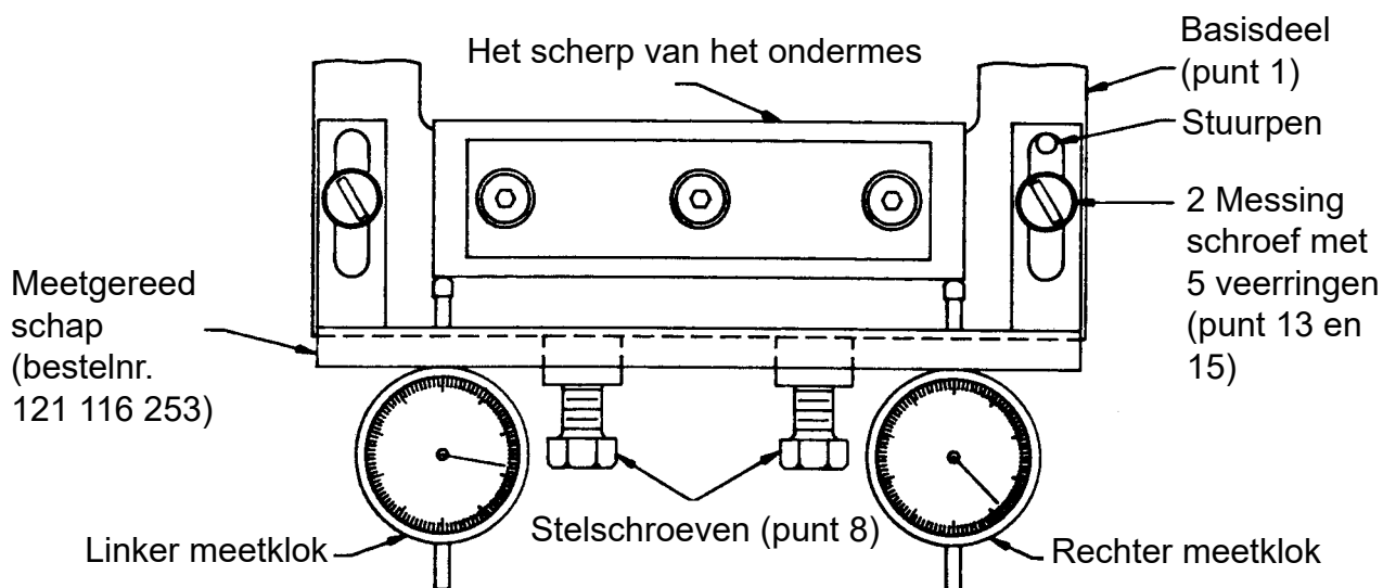
FIG. 8: Multicutter van boven af gezien
