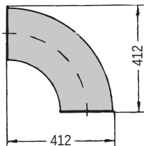
90° bend, galv. R = 300 122 050 116
