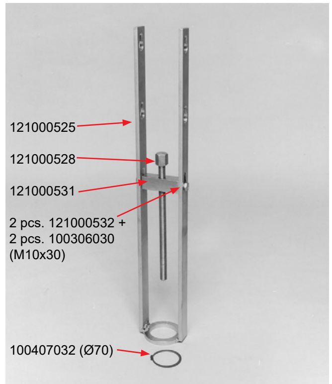
TRL/SUC 500 + 700 + 1000 + SupraVac 2000
