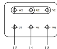
Connexion en estrella
