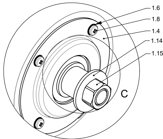
DETAIL B (1 : 2)
