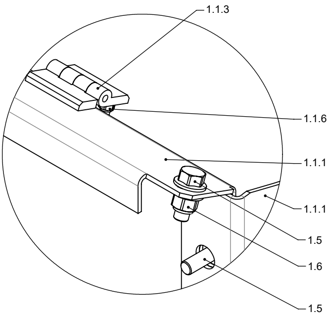
DETAIL B (1 : 2)
