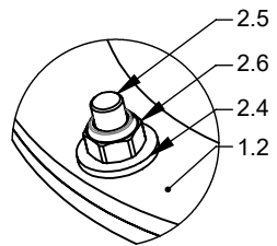
DETAIL D (1 : 2)
