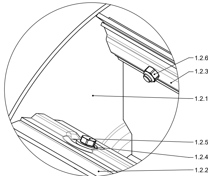
DETAIL D (1 : 2)
