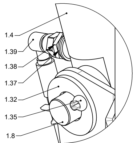
DETAIL B (1 : 2)
