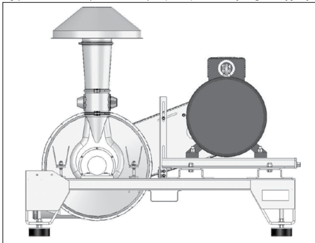
Typ 2: OK200 (ø200 mm) z przepustnicą regulacyjną
