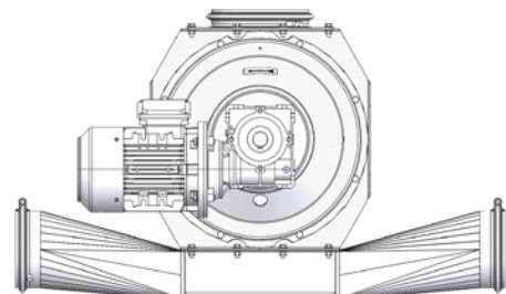
CAD 40 avec sortie horizontales OK160
