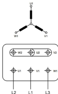
Connexion en étoile
