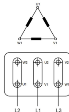
Connexion en triangle
