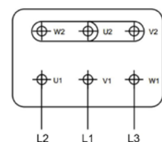
Stjerneforbindelse
