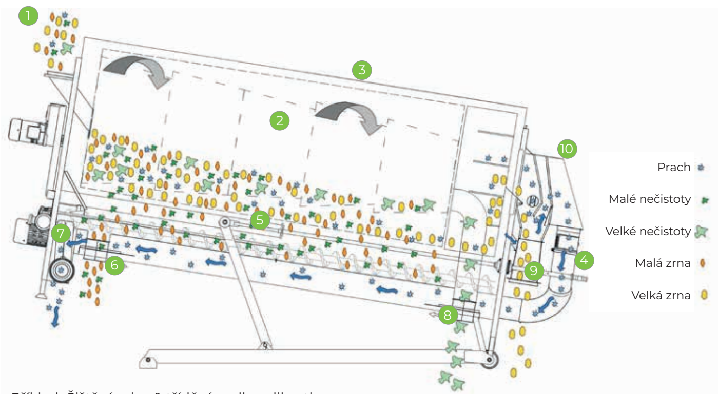
Příklad: Čištění osiva & třídění podle velikosti zrna
