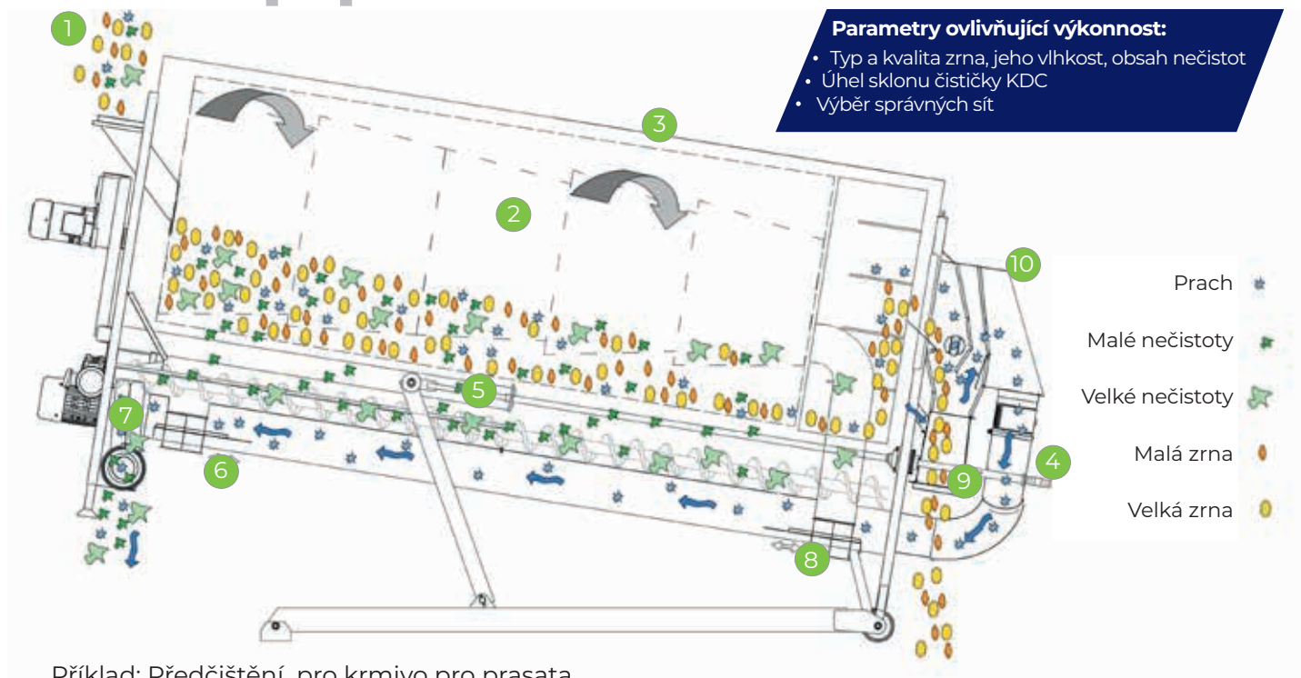
Příklad: Předčištění pro krmivo pro prasata
