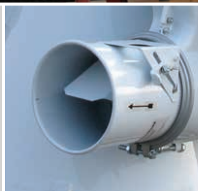
Klapka regulace vzduchu pro nastavení sací síly ventilátoru
